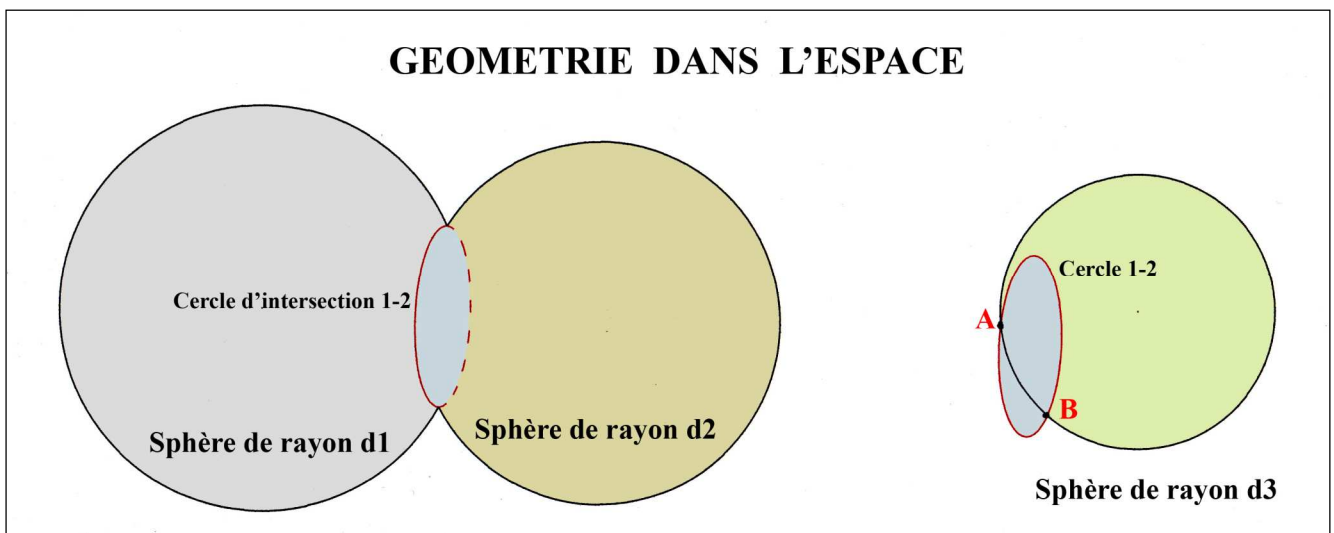
Principe de la multilatération. Avec 3 distances d_1 , d_2 , d_3 , on obtient deux solutions A et B, faciles à trancher.
